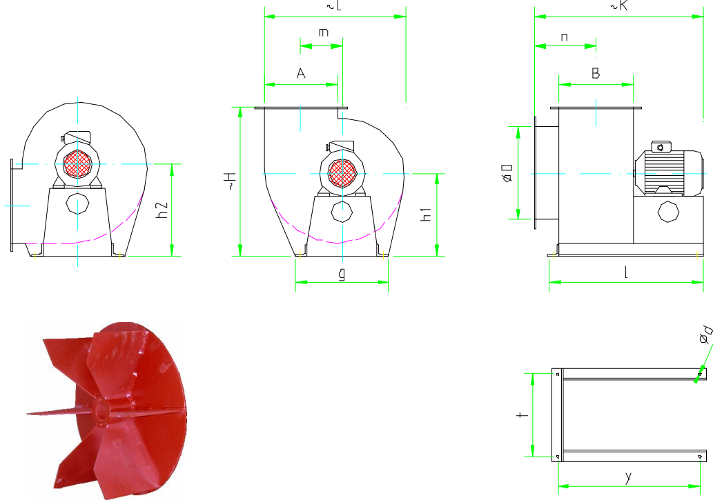
EBAT TABLOSU (1400 rpm)
